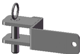
1/2 bride nue pour poteau carré de 80 veau code: 5726000
